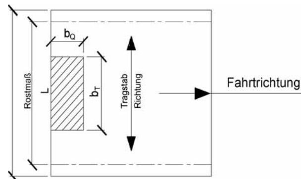
Bild 1 – Schweißpressroste (Lastanordnung 1)
