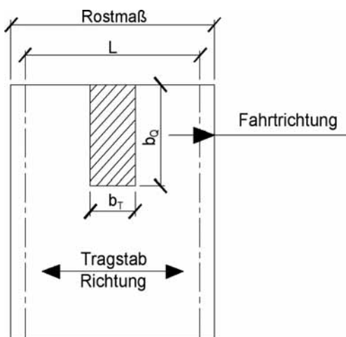
Bild 2 Schweißpressroste (Lastanordnung 2)
