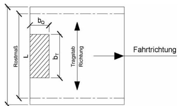
Bild 3 – Pressroste (Lastanordnung 1)
