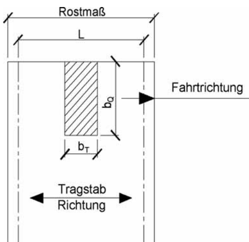
Bild 4 – Pressroste (Lastanordnung 2)
